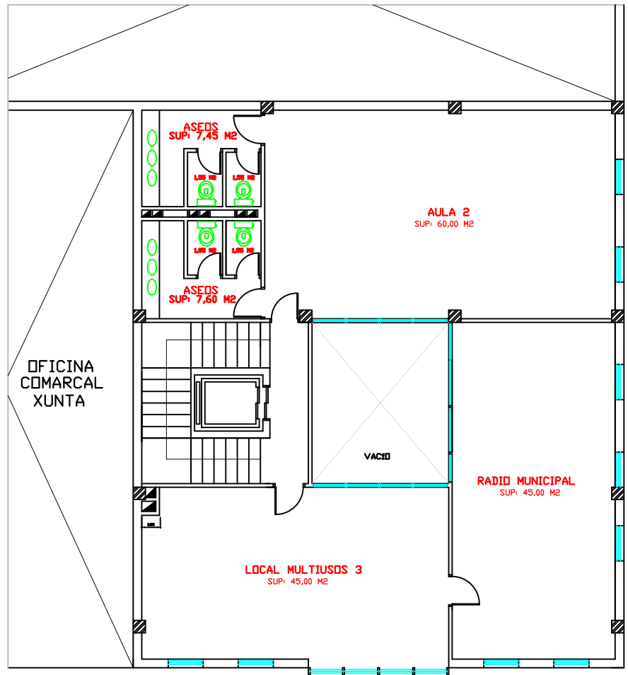
PLANTA SEGUNDA
